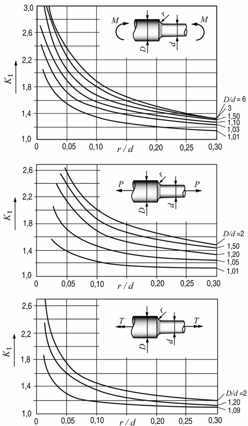
Kuva 1 Akselin olakkeen lovenmuotolukuja taivutuksessa, aksiaalisessa kuormituksessa ja väännössä
